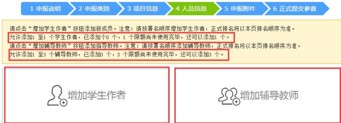
图 4-1 人员信息
