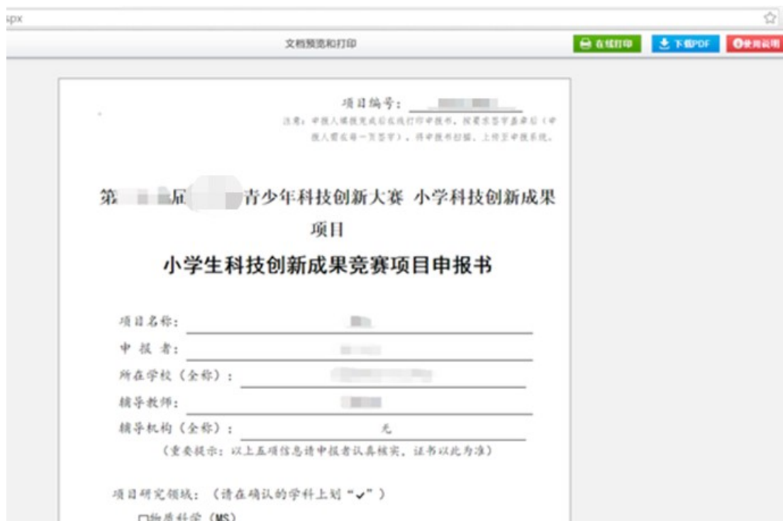
图 6-3 打印页面
